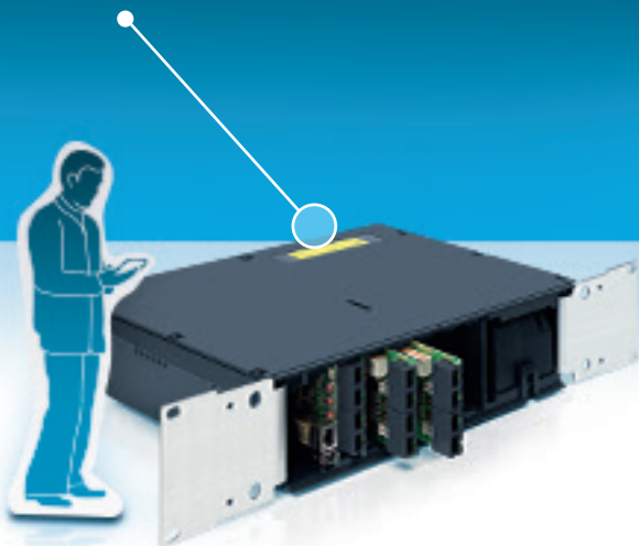
COMcompact 5000 und 5000R ohne die Abdeckung für Anschlüsse und Erweiterungsmodule
